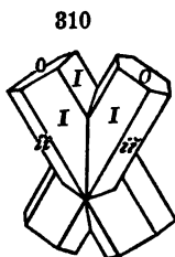
Staurolite.
